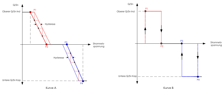
Abbildung 8-3 Q(U)-Kurve
