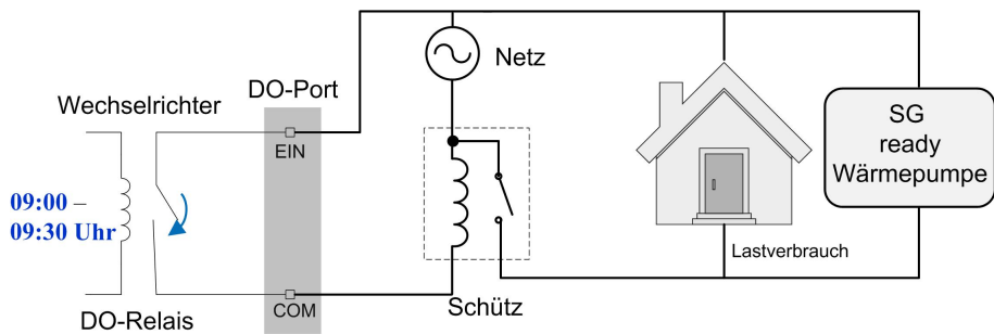
Abbildung 8-21 DO-Betrieb im Zeitplan-Modus
