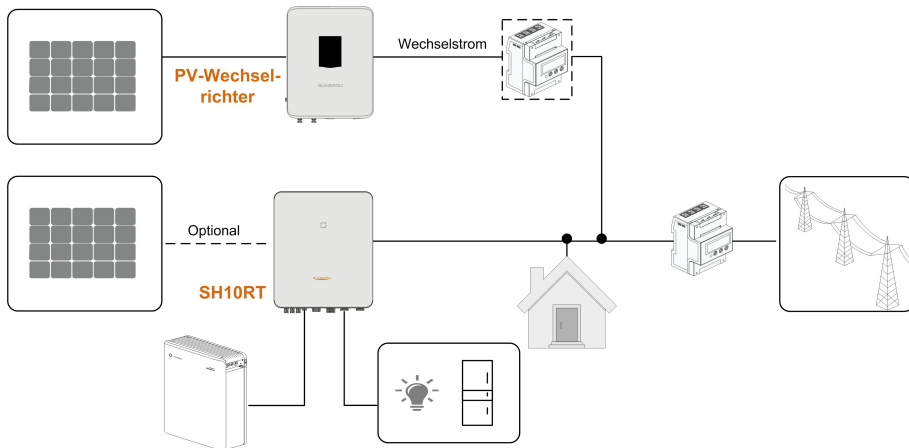
Abbildung 2-4 Nachrüstung einer vorhandenen PV-Anlage
