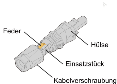
Abbildung 6-4 Komponenten des SUNCLIX-Steckers
