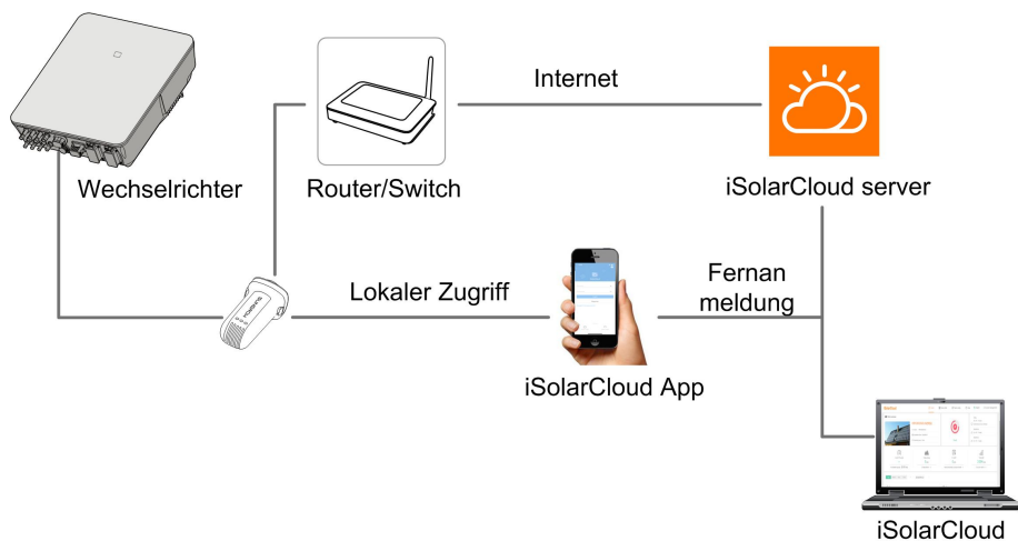
Abbildung 6-3 WLAN-Verbindung mit dem WiFi-Modul
