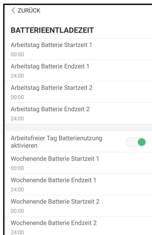
Abbildung 8-18 Batterieentladezeit
