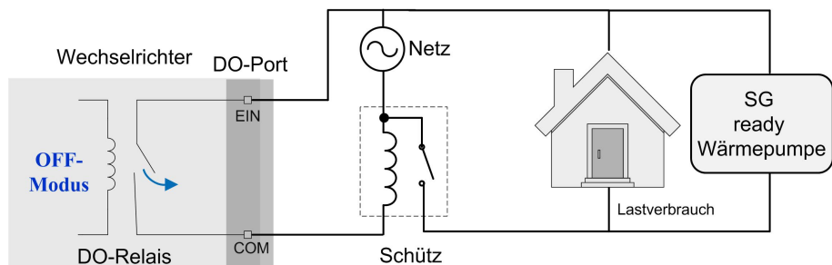
Abbildung 8-22 DO-Betrieb im Schalter-Modus
